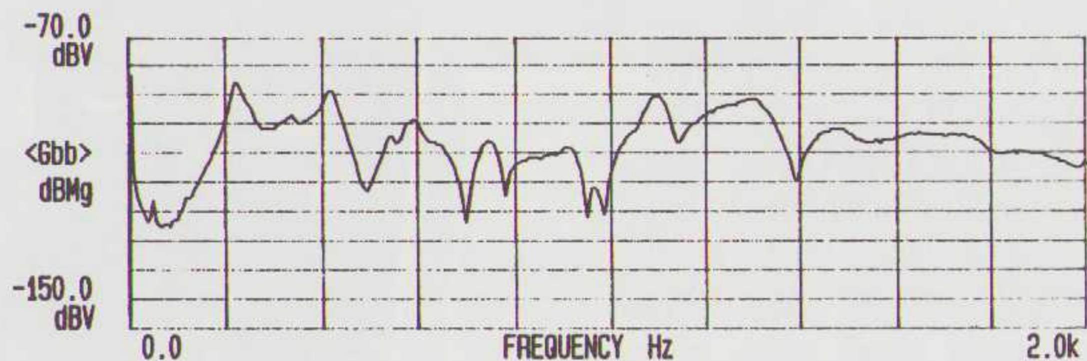
Paneelresonantie van het eerste model van de PMR luidspreker
